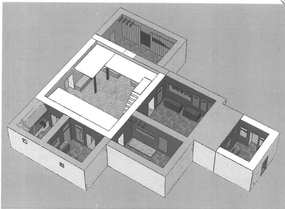
Distribución de elementos planta baja
